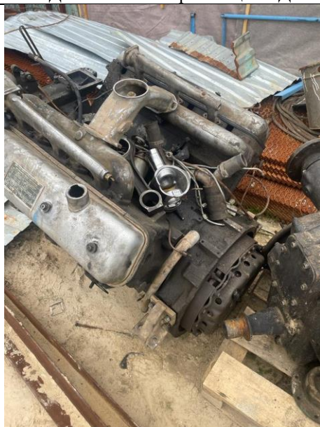
Дизельная электростанция ЭД200-Т400-1РН в утепленном контейнере типа "Север" 025
